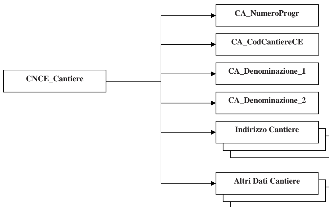
Figura 4: struttura Cantiere
