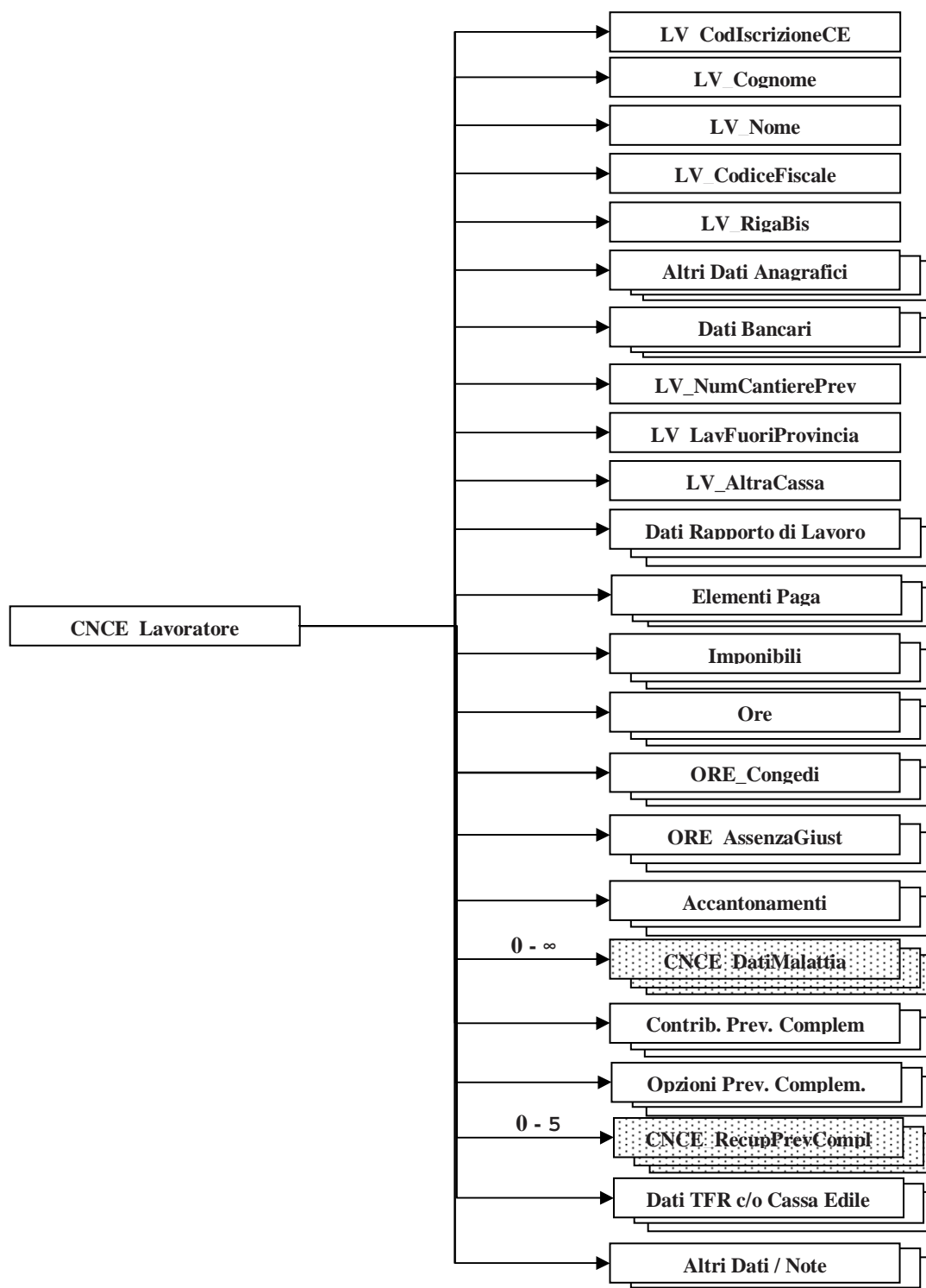
Figura 5: struttura Lavoratore
