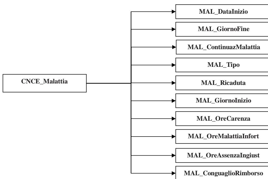
Figura 6: struttura Malattia
