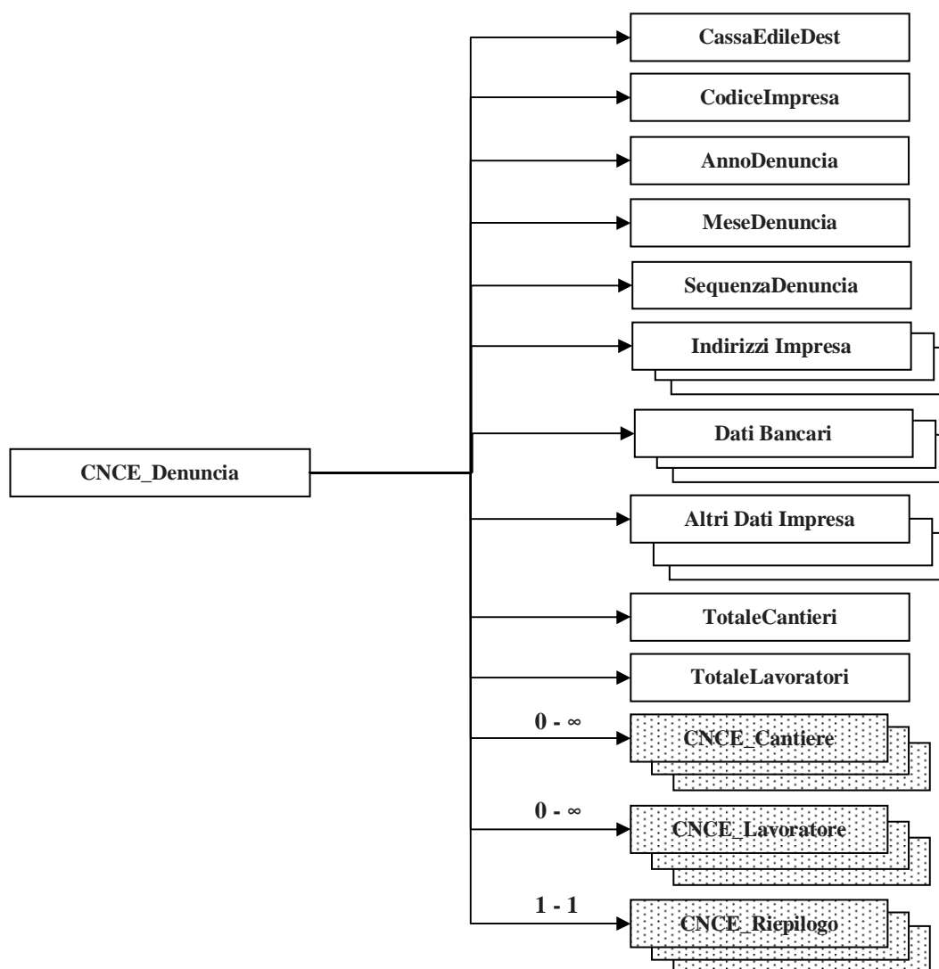
Figura 3: struttura Denuncia
