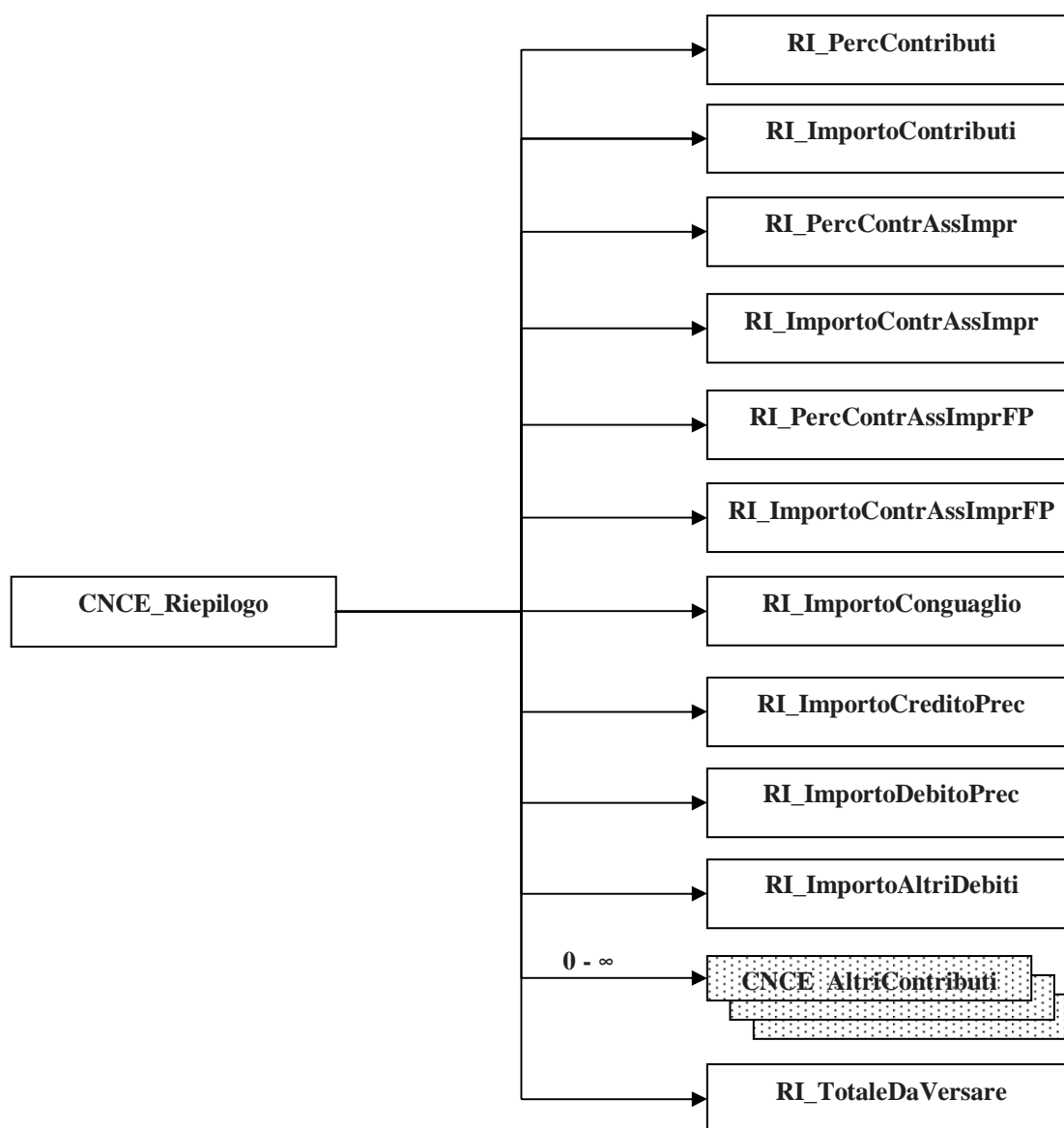
Figura 8: struttura Riepilogo
